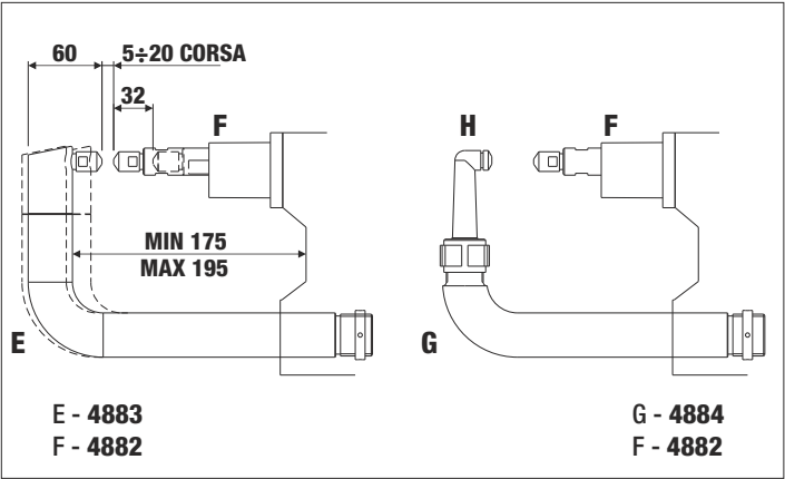
Caratteristiche bracci con art. 3323 Arms features with item 3323 Caractéristiques des bras avec art. 3323 Daten der Arme mit Art. 3323 Caracteristicas brazos con art. 3323
