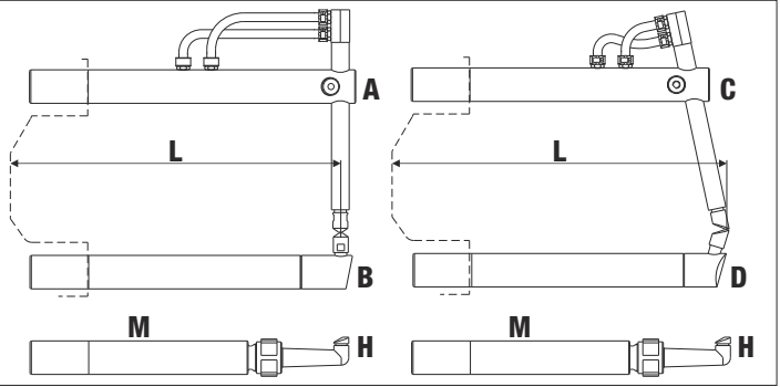
BRACCI PER ART. 3324 / ARMS FOR ITEMS 3324 / BRAS POUR MODELES 3324 / ARME ZU TYPEN 3324 / BRAZOS PARA ART. 3324
