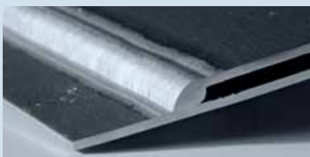
Saldatura AC-MIG con VARIGON® He15S su lamiere di spessore 1 mm e gap 1,5 mm
